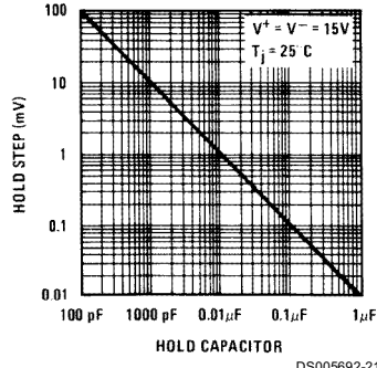
Hold Step
