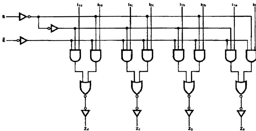
'S157 • 'LS157
