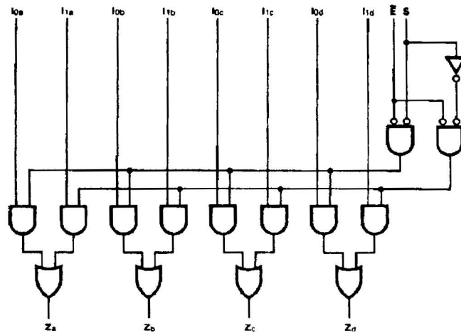
'S157 • 'LS157
