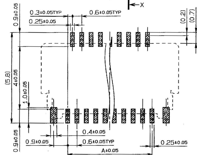
基板取付寸法 MOUNTING LAYOUT
