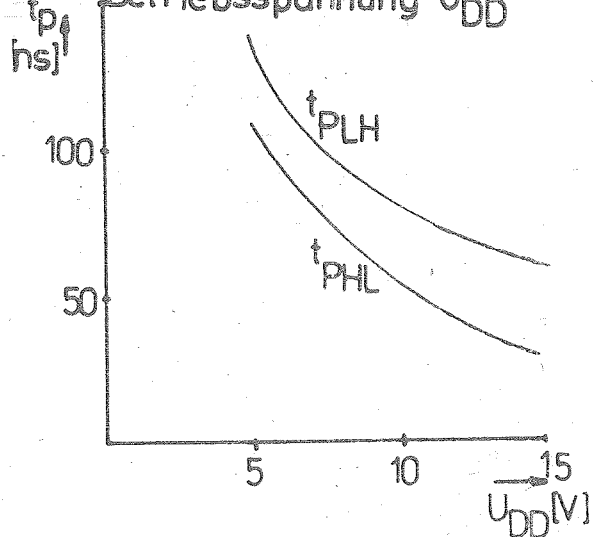
Funktion Gatterlaufzeit / Betriebsspannung U_{DD}
