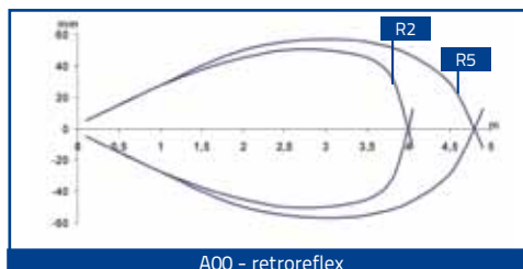
A00 - retroreflex
