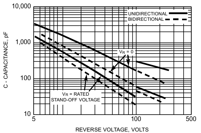
FIG. 6 - CAPACITANCE
