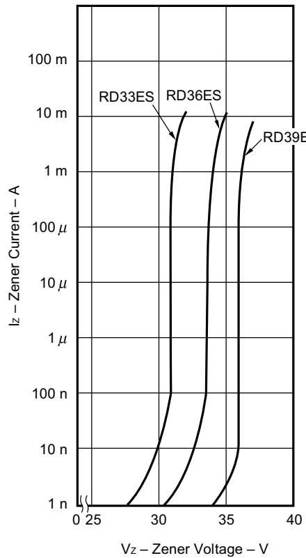
Fig. 5 ZENER CURRENT vs. ZENER VOLTAGE
