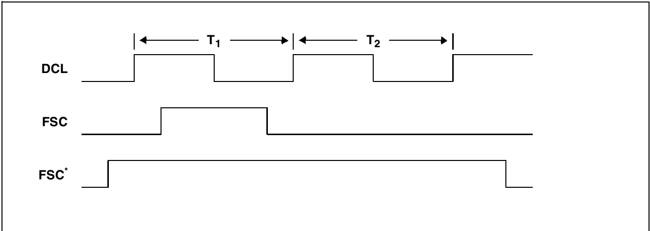
Figure 39 IOM ® -2 Interface - Frame Start
