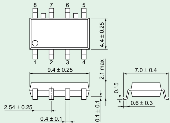
2.54SOP8
