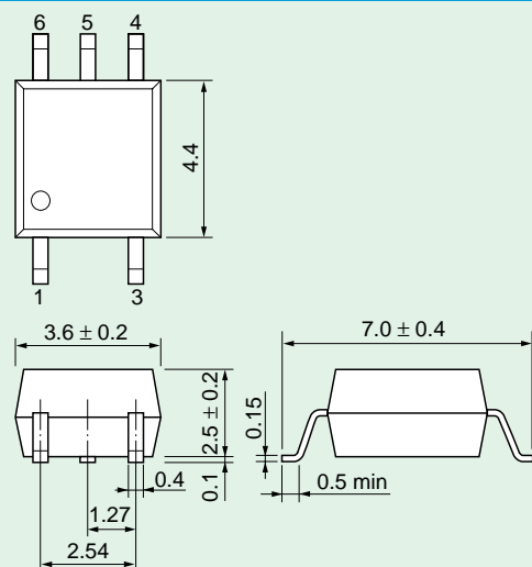
5-pin MFSOP6
