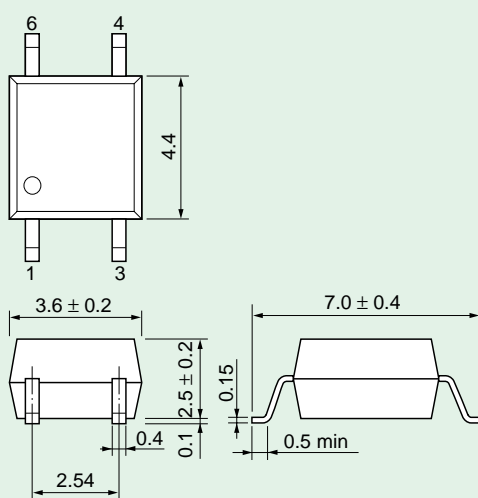
4-pin MFSOP6
