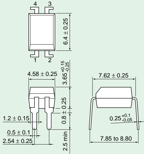
DIP4 (LF2)
