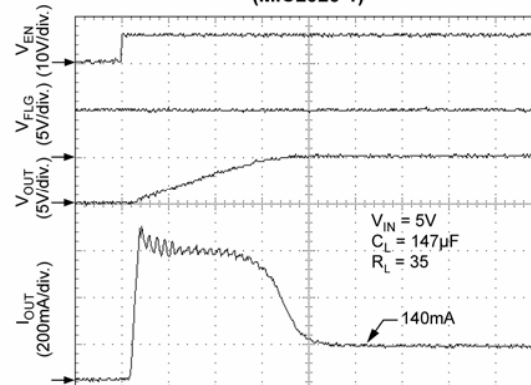
Turn-On (MIC2026-1)
