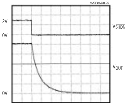
500 \mu s /div NO LOAD
