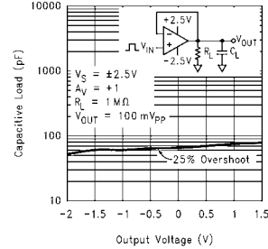
Output Voltage (V) DS100060-47
