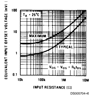
Offset Error
