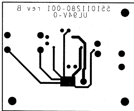
Bottom Layer
