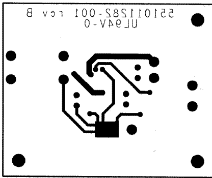
Bottom Layer
