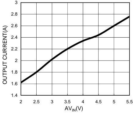
Maximum Sinking Current vs AV IN (V DDQ =2.5V)
