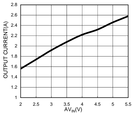
Maximum Sinking Current vs AV IN (V DDQ =1.8V)
