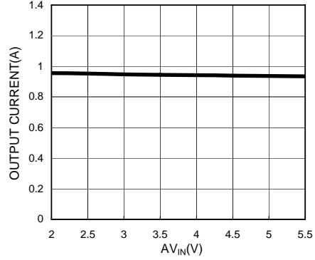
Maximum Sourcing Current vs AV IN (V DDQ =1.8V, P VIN =1.8V)
