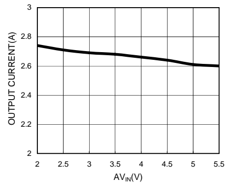
Maximum Sourcing Current vs AV IN (V DDQ =1.8V, P VIN =3.3V)
