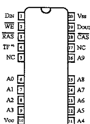
20 (26) SOJ
