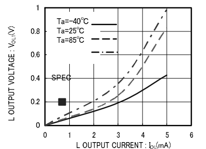
Fig.5 'L' output voltage V_{OL} ( V_{CC}=1.7V )
