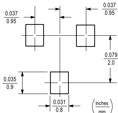
SOT-23
