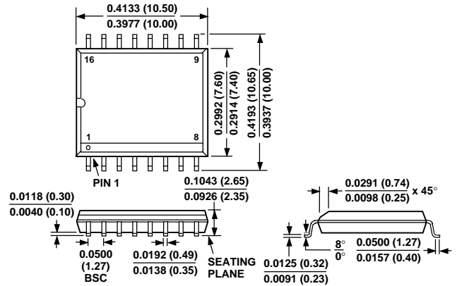
SOIC (R-16)
