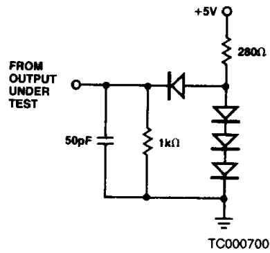
TTL Outputs
