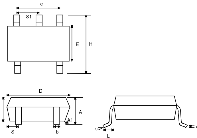
SOT-23-5
