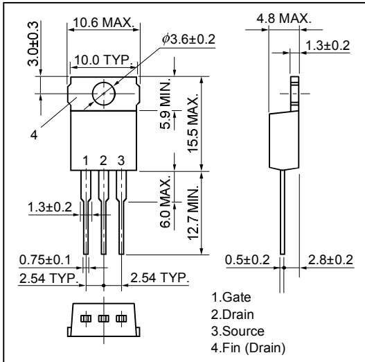
1) TO-220AB (MP-25)
