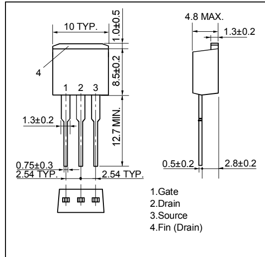
2) TO-262 (MP-25 Fin Cut)
