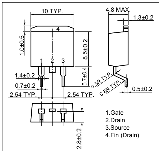
3) TO-263 (MP-25ZJ)
